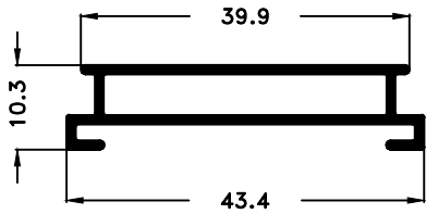
PM-1524 0,314 Kg/m
