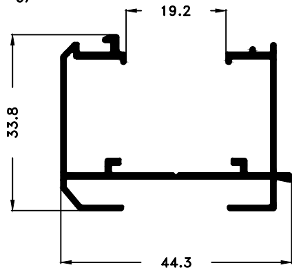
PM-5762 0,489 Kg/m
