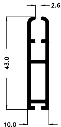
PM-4622 0,448 Kg/m
