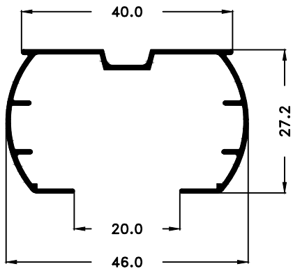
PM-0765 0,279 Kg/m
