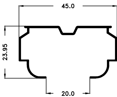
PM-5239 0,236 Kg/m
