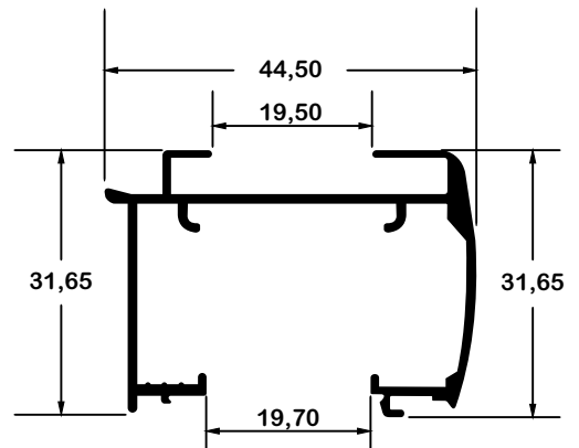
PM - 4510 0,446 Kg/m
