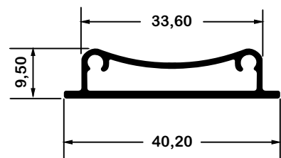
PM - 1953 0,316 Kg/m
