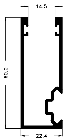
PM-5298 0,688 Kg/m
