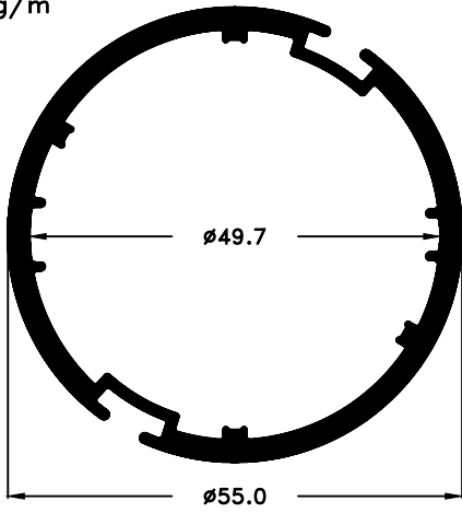
PM-5562 1,219 Kg/m
