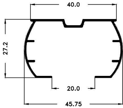
PM-1669 0,260 Kg/m
