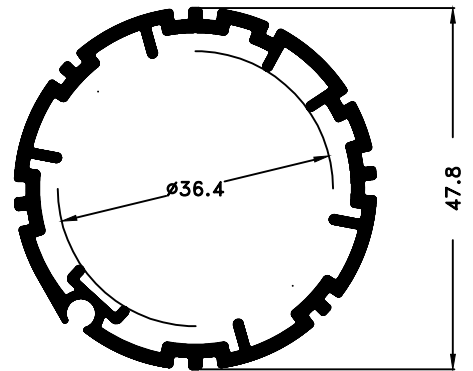
PM-2312 0,869 Kg/m
