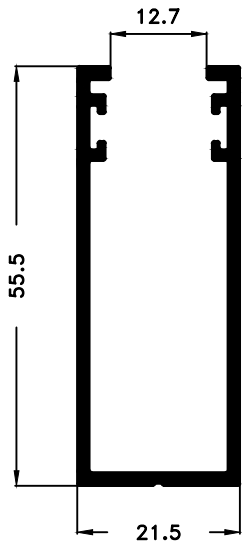
PM-1304 0,642 Kg/m
