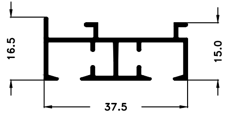
PM-1415 0,320 Kg/m
