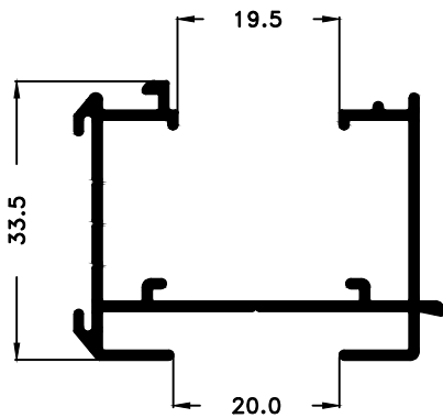
PM-1654 0,492 Kg/m
