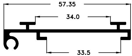
PM-4587 0,342 Kg/m
