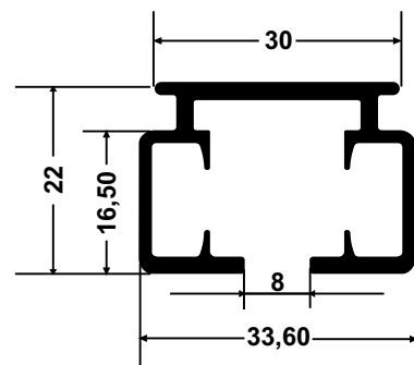
PM-2730 0,528 Kg/m
